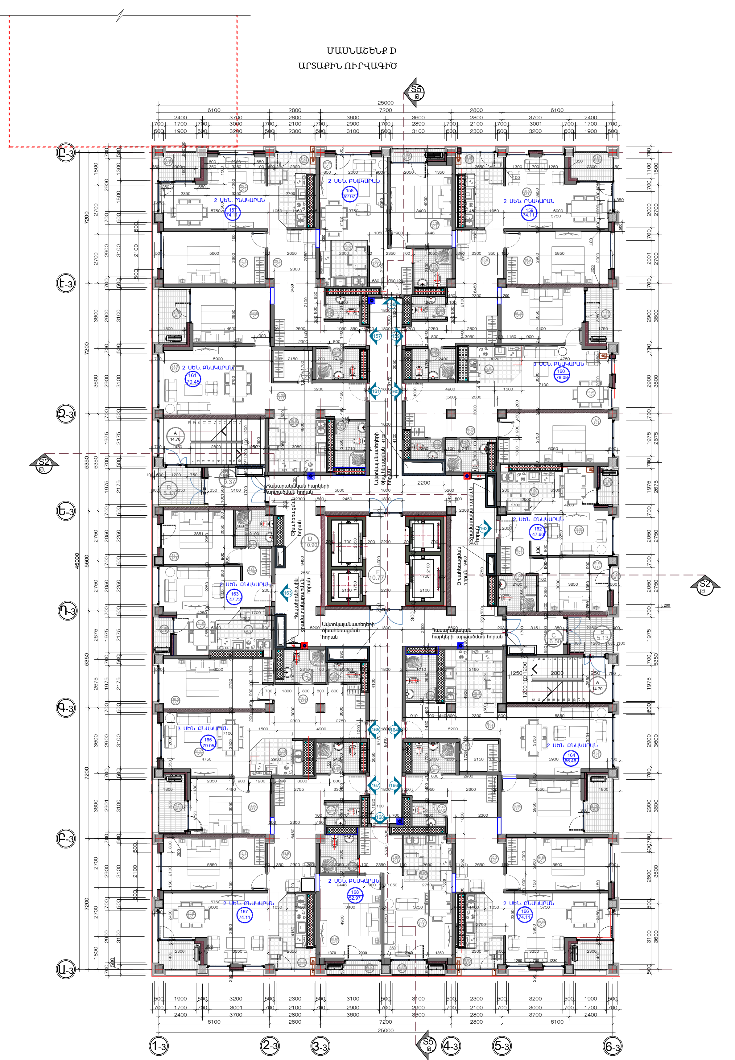
ՀԱՐԿԻ ՀՆԱՍԿԱԳԻԾ /ՆԻՇ. 49.500 / Մ: 1/125 ՄԱՍՆԱՇԵՆՔ A
