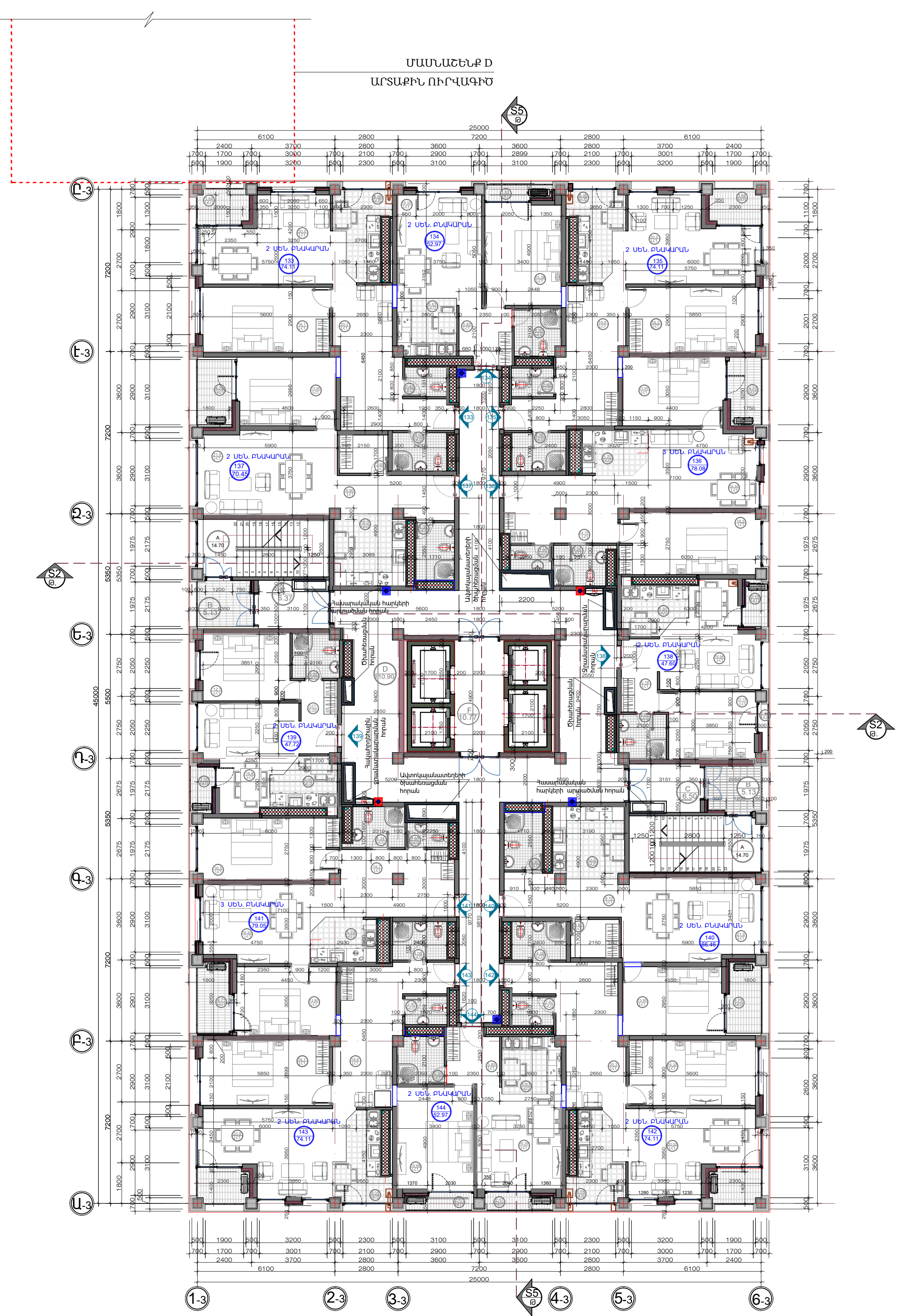
ՀԱՐԿԻ ՀՍԱԿԱԳԻԾ /ՆԻՇ. 42.900 / Մ: 1/125 ՄԱՍՆԱՇԵՆՔ A
