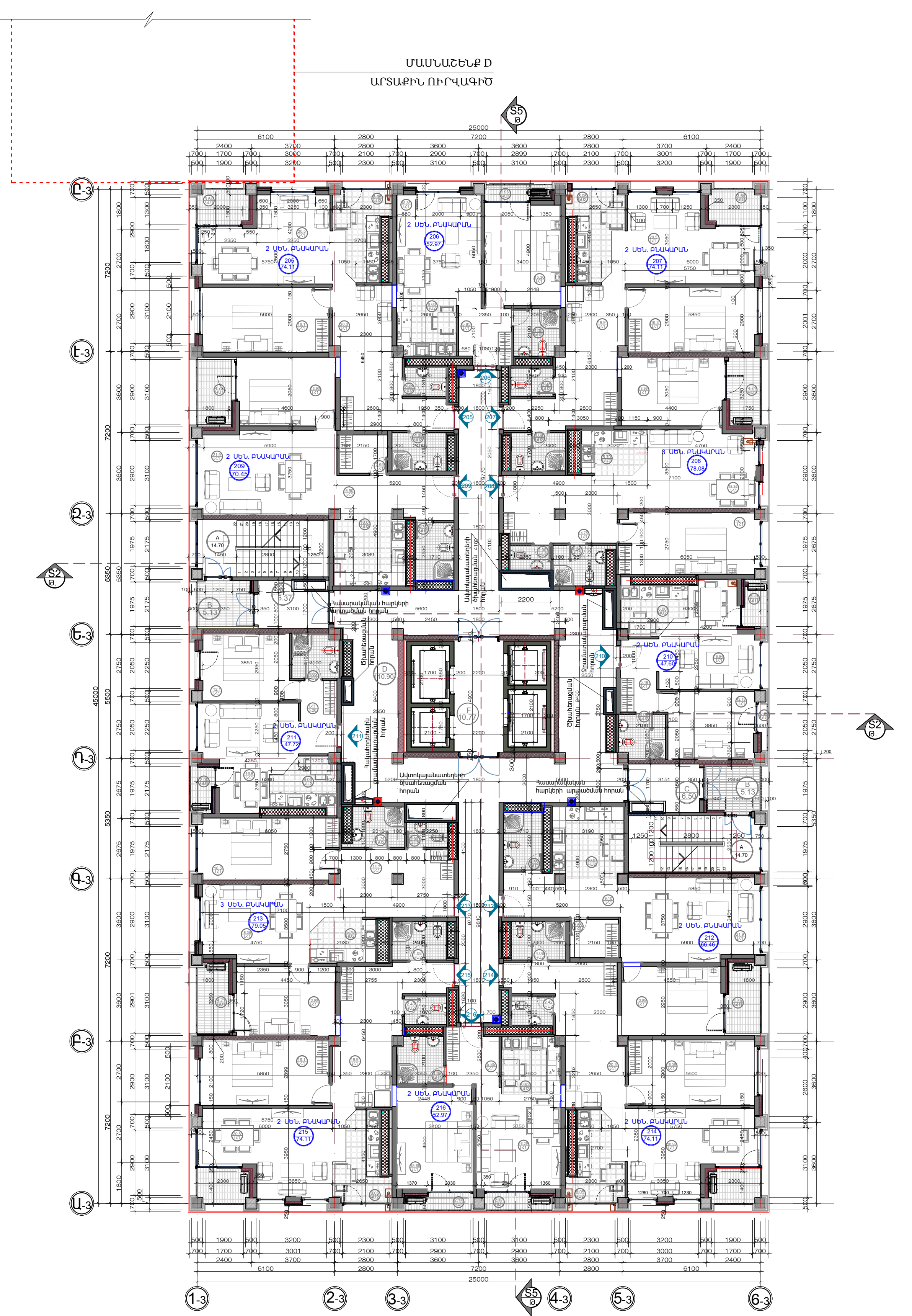
ՀԱՐԿԻ ՀՍԱԿԱԳԻԾ /Ն.Բ. 62.700 / Մ: 1/125 ՄԱՍՆԱՇԵՆՔ A
