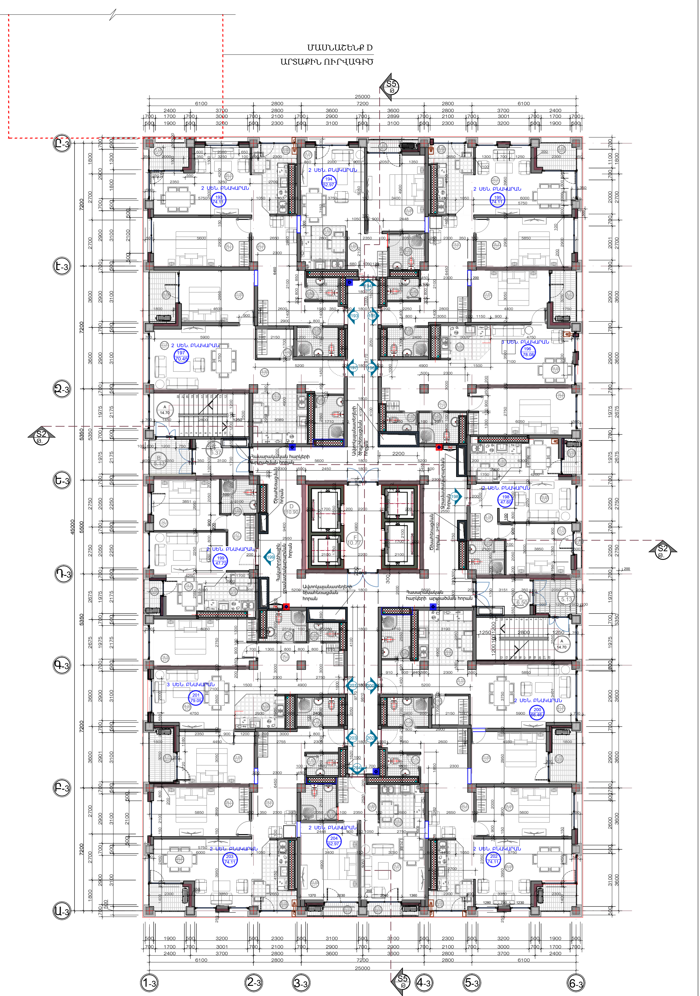
ՀԱՐԿԻ ՀՆԱՍԿԱԳԻՏ /Ն.Ը. 59.400 / Մ: 1/125 ՄԱՍՆԱՇԵՆՔ A
