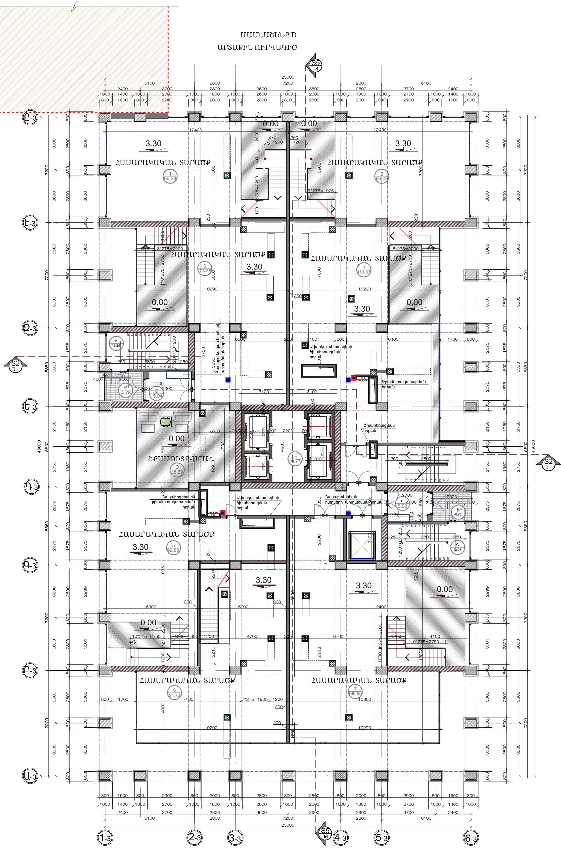
ՀԱՐԿԻ ՀԱՍՏԱՐԱԿԱՎԱՆ ԴՐ. 3.300/ Մ: 1/125 ՄԱՍՆԱՇԵՆՔ A
