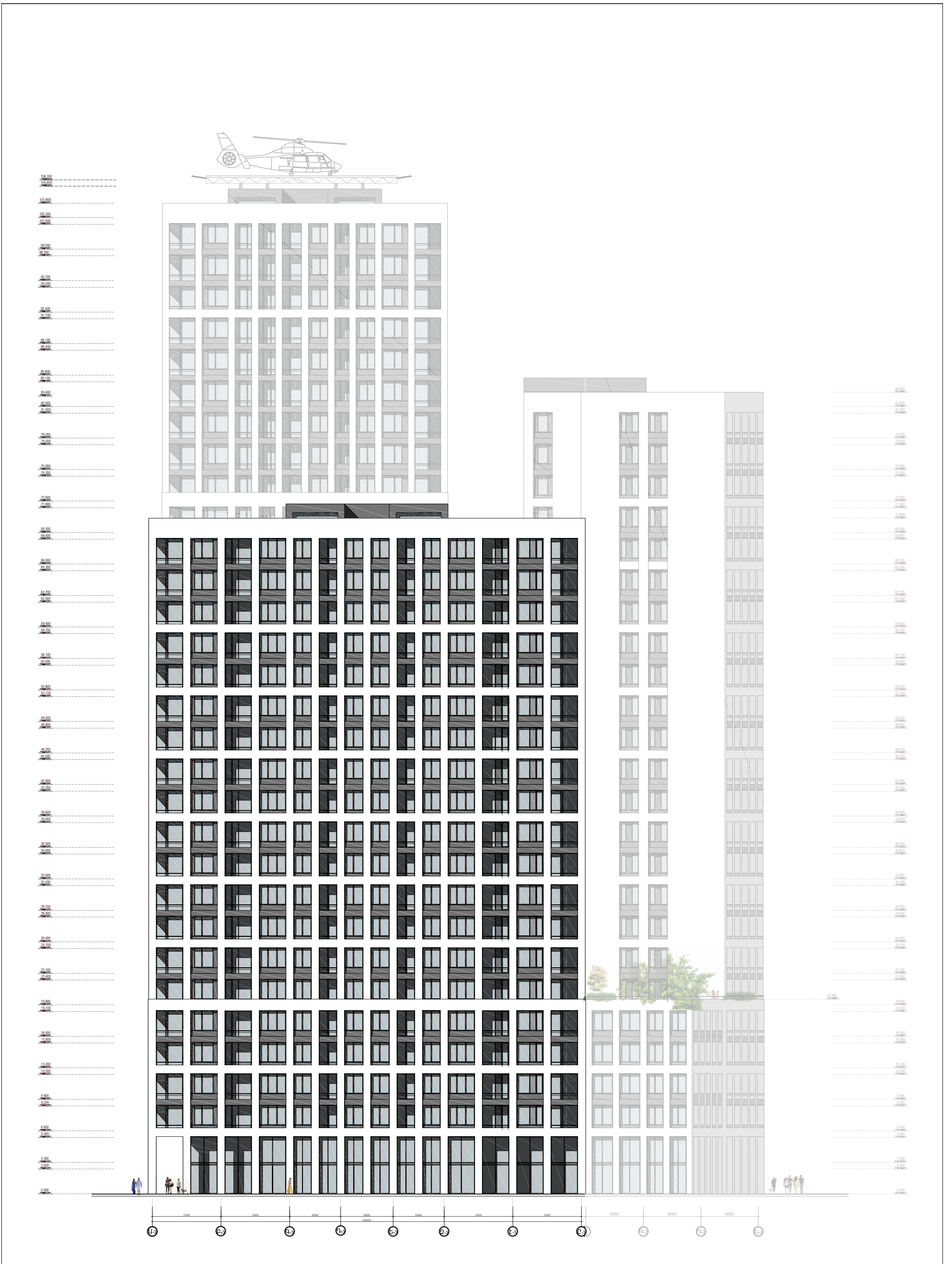
ՃԱԿԱՏ ԸՍՏ Ա-3 ԵՎ Ը-3 ԱՌԱՆՑՔՆԵՐԻ Մ 1:250
