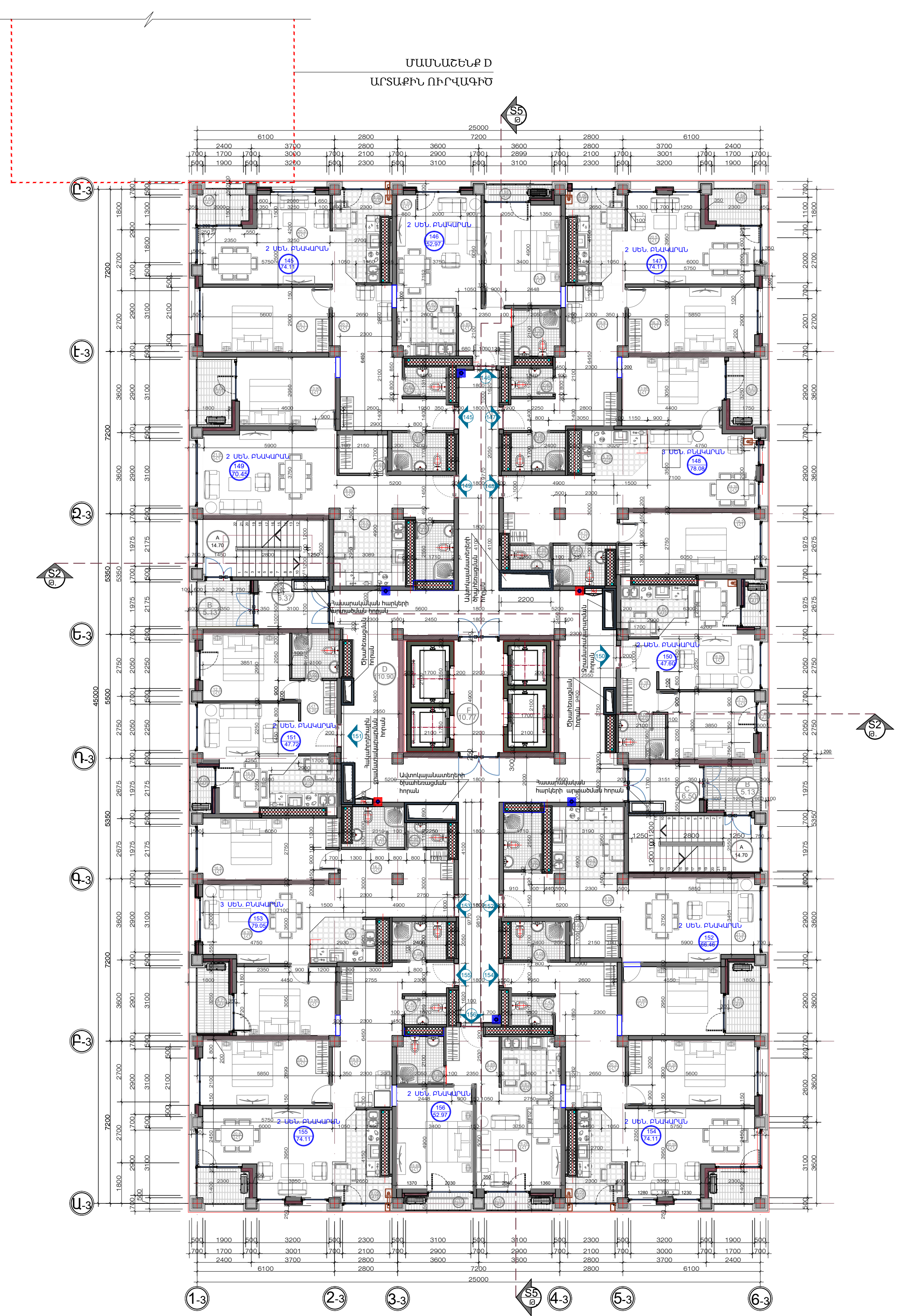
ՀԱՐԿԻ ՀՍԱԿԱԳԻԾ /Ն.Ը. 46.200 / Մ: 1/125 ՄԱՍՆԱՇԵՆՔ A
